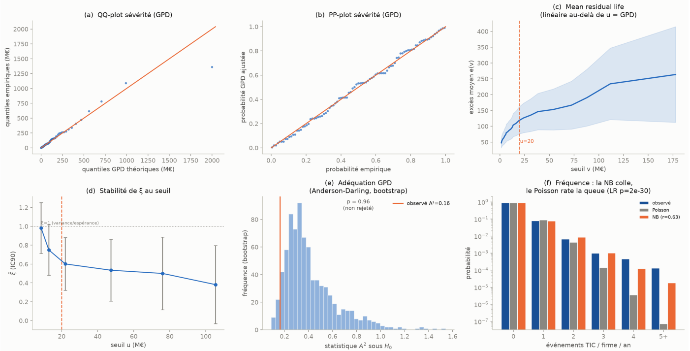
Figure 5.4. Validation du socle. (a-b) QQ-plot et PP-plot de la sévérité contre la GPD ajustée. (c) vie résiduelle moyenne, linéaire au-delà de u . (d) stabilité de \xi au seuil. (e) test d'Anderson-Darling, loi nulle par bootstrap paramétrique et statistique observée ( p = 0,96 ). (f) adéquation de la fréquence : la NB colle aux comptes firme-année, le Poisson rate la queue. Source : script 47.
