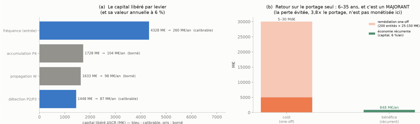
Figure C.9. Le ROI de la conformité. (a) le capital libéré par levier, classé, avec sa valeur annuelle à 6 % (bleu : calibrable, gris : borné). (b) coût de remédiation one-off contre économie récurrente de portage du capital ; le retour sur le portage seul est de 6 à 35 ans, et c'est un majorant , la perte évitée n'étant pas monétisée ici. Sources : scripts 50 et 67.
