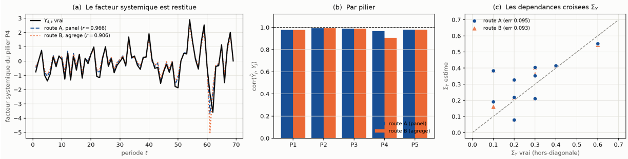
Figure 7. (a) Le facteur systémique du pilier P4 est restitué par les deux routes. (b) Par pilier, la corrélation dépasse 0,90 partout. (c) Les dépendances croisées \Sigma_Y sont retrouvées avec une erreur absolue moyenne de 0,09.
