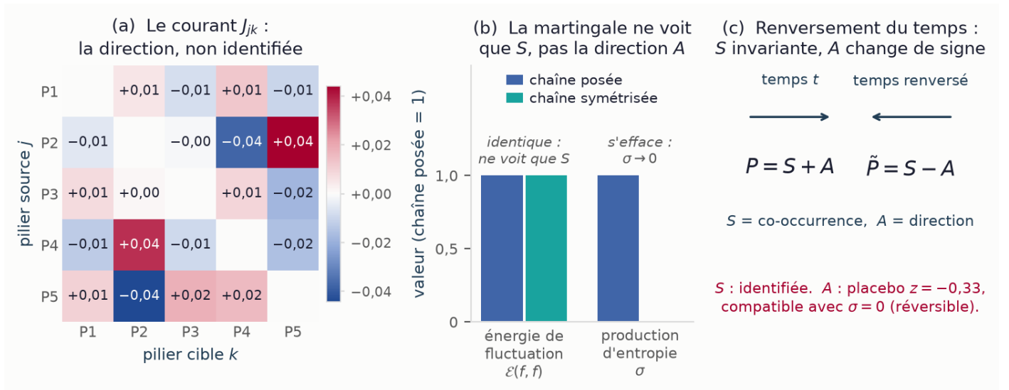
Figure 8.1. La direction A comme courant irréversible, et pourquoi la donnée ne peut pas la voir. (a) le courant J_{jk} = \pi_j P_{jk} - \pi_k P_{kj} est non nul : le modèle porte bien une direction. (b) l'énergie de fluctuation, c'est-à-dire la variation quadratique de la martingale, est identique pour la chaîne posée et pour sa symétrisée : elle ne voit que S . La production d'entropie, elle, s'efface à la symétrisation. (c) le renversement du temps laisse S intacte et retourne le signe de A . C'est la raison de principe pour laquelle une statistique de co-occurrence, invariante par renversement, ne peut pas identifier un courant qui change de signe sous ce renversement.
