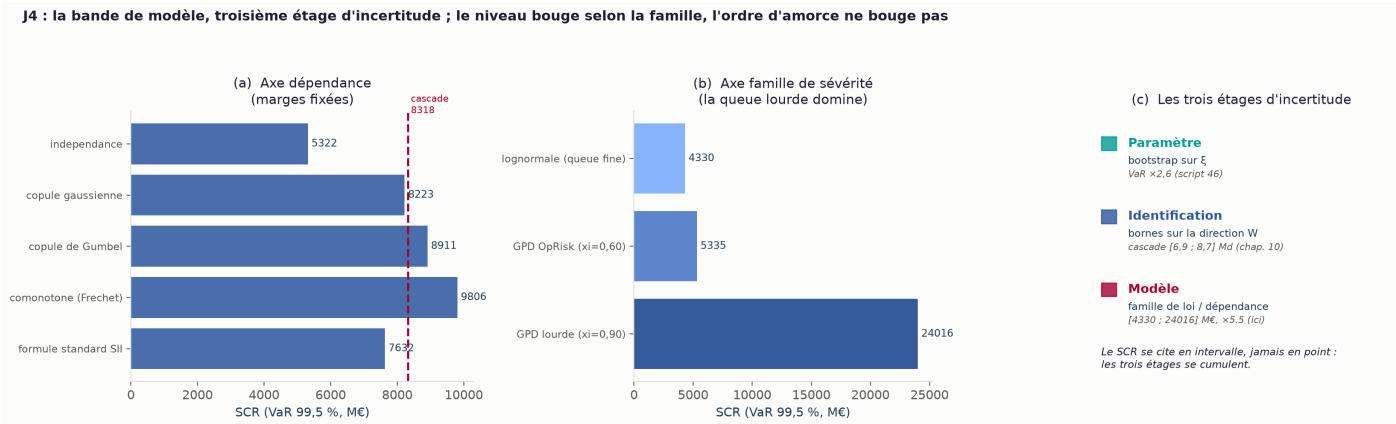
Figure 11.1. La bande de modèle, troisième étage d'incertitude. (a) axe dépendance, à marges fixées : la cascade se place entre les copules gaussienne et de Gumbel, dans une bande [5,3 ; 9,8] Md€. (b) axe famille de queue : la queue lourde domine l'incertitude ( \times 5,5 ). (c) les trois étages (paramètre, identification, modèle) tels que le script les cumule ; la bande reportée par le mémoire n'en retient que les deux premiers, le troisième étant publié comme axe de sensibilité (§11.2.1). Source : script 48.
