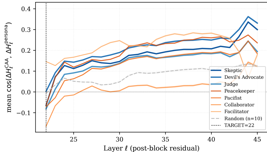
Gemma 2 27B
