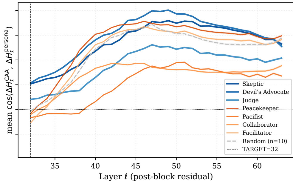
Qwen 3 32B
