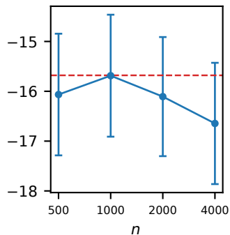
Rademacher, p=5
