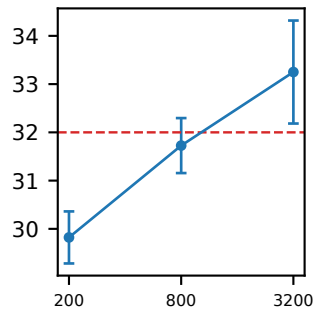
Rademacher, p=5
