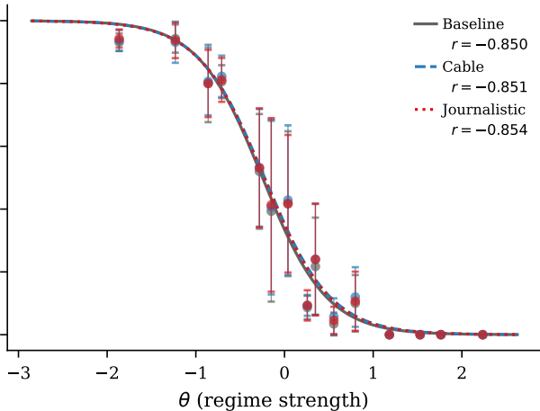
Llama 3.3 70B
