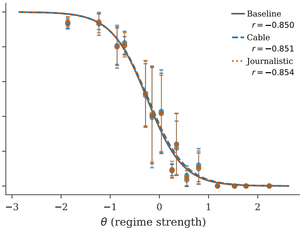
Llama 3.3 70B
