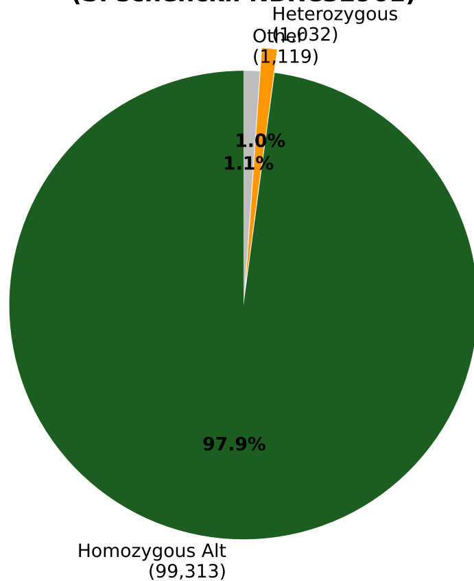
A. Variant Zygosity ( S. schenckii NBRC32961)
