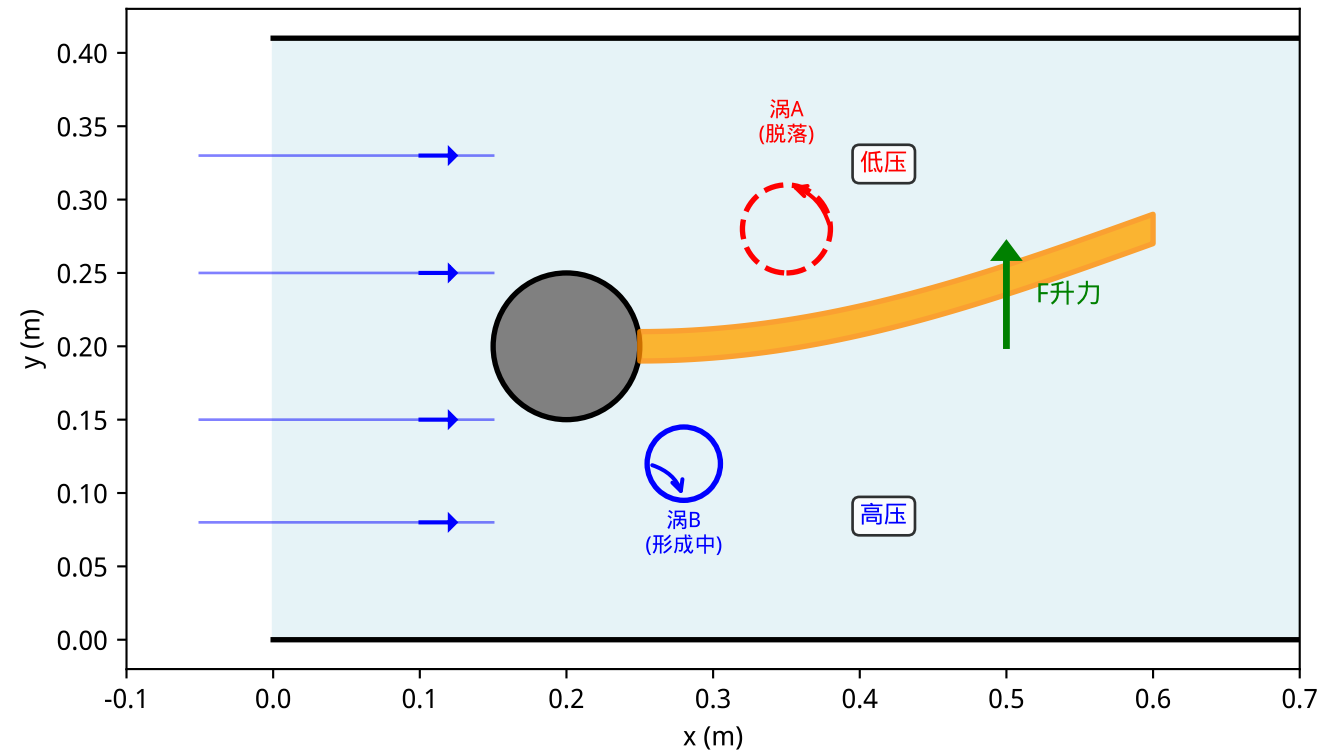
(a) 板向上运动：上方涡脱落，产生向上升力
