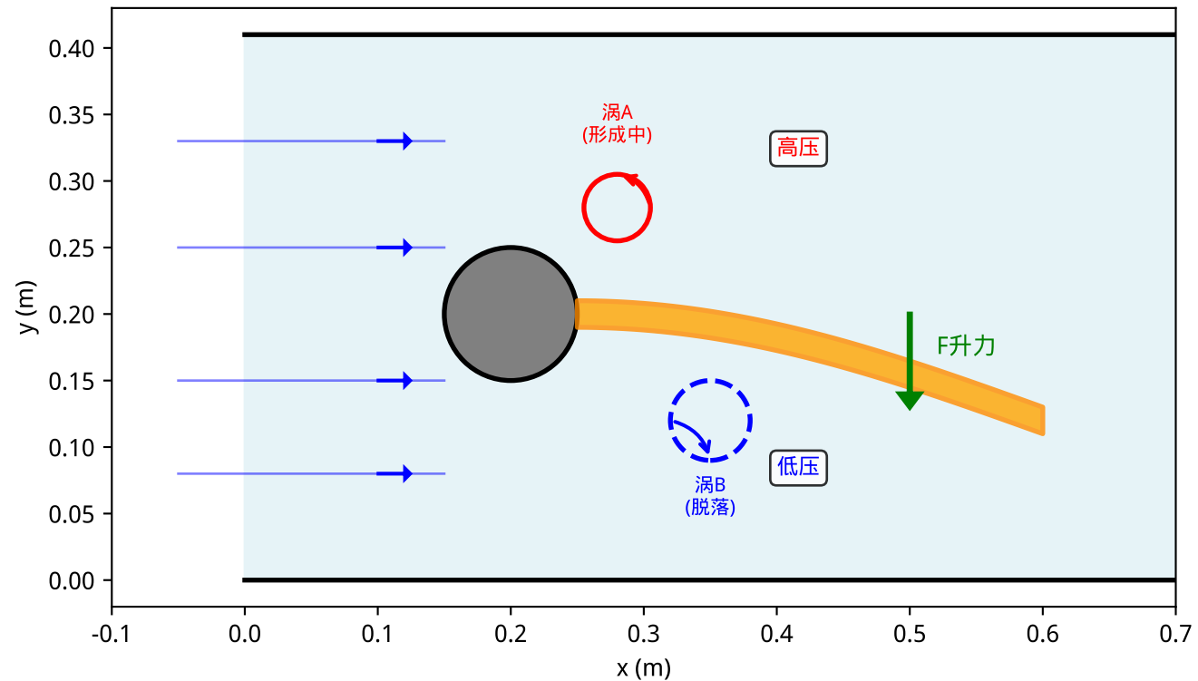
(b) 板向下运动：下方涡脱落，产生向下降力
