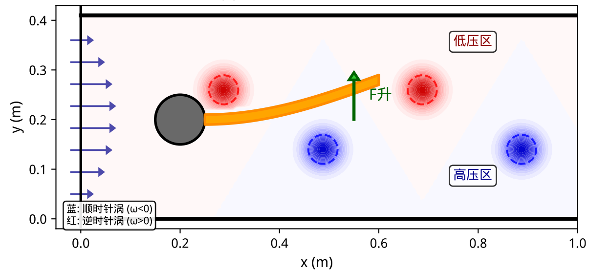
(a) 板向上运动：上方涡脱落
