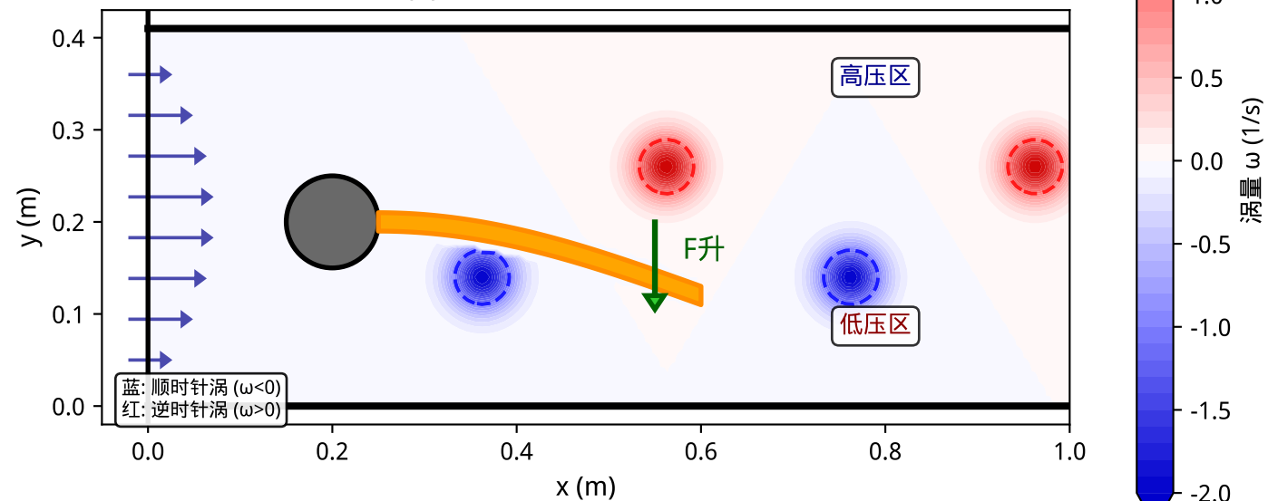
(b) 板向下运动：下方涡脱落
