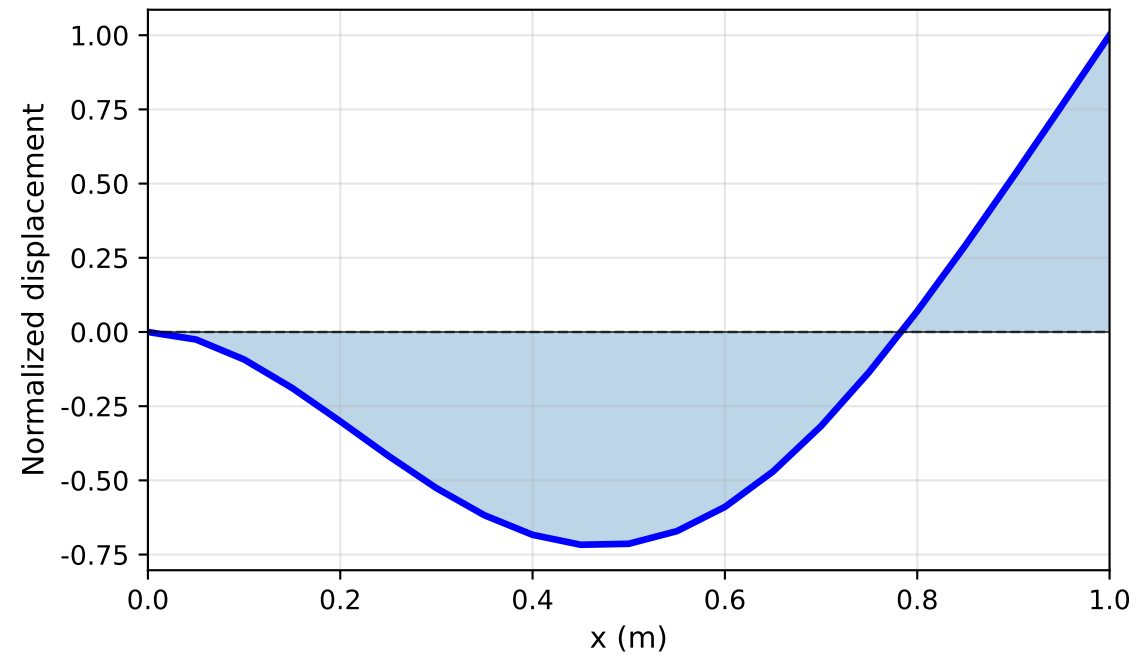
Mode 4: f_4 = 574.64 Hz
