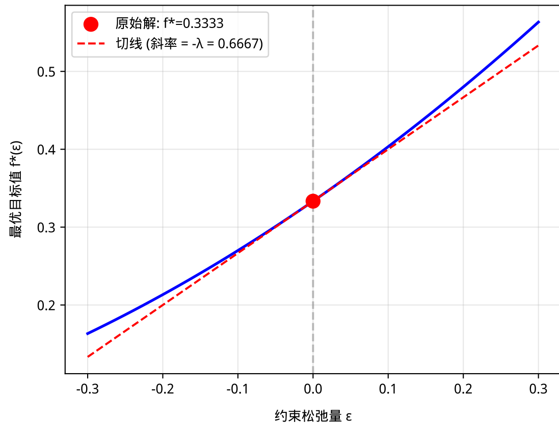
影子价格: \lambda = df^*/d\varepsilon (最优值对约束的敏感度)
