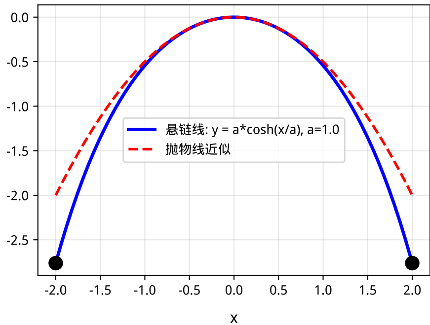
悬链线 vs 抛物线 (a=1)
