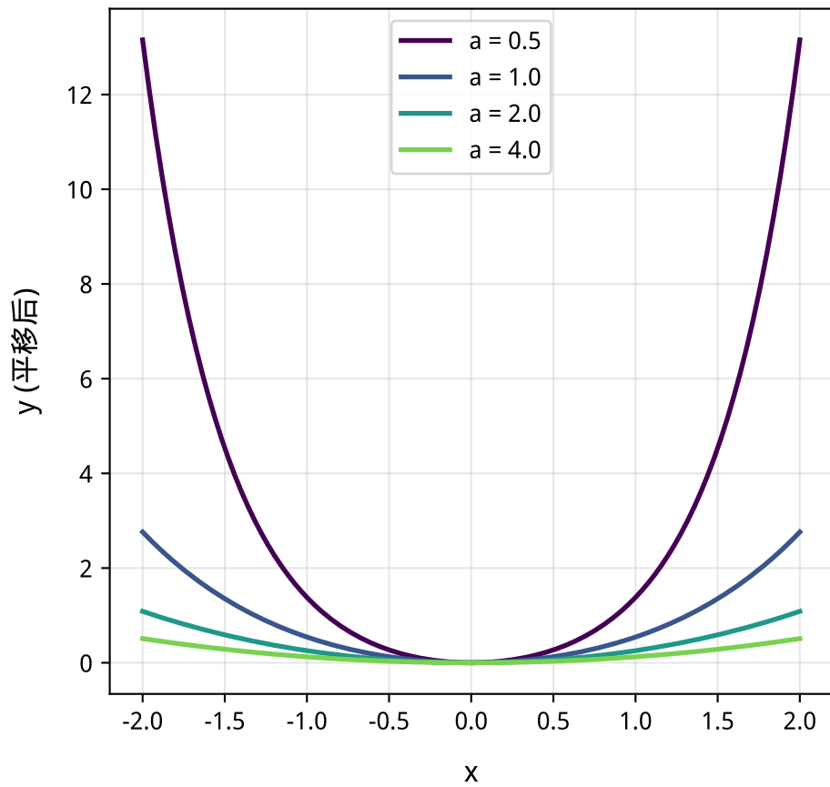
不同参数a的悬链线
