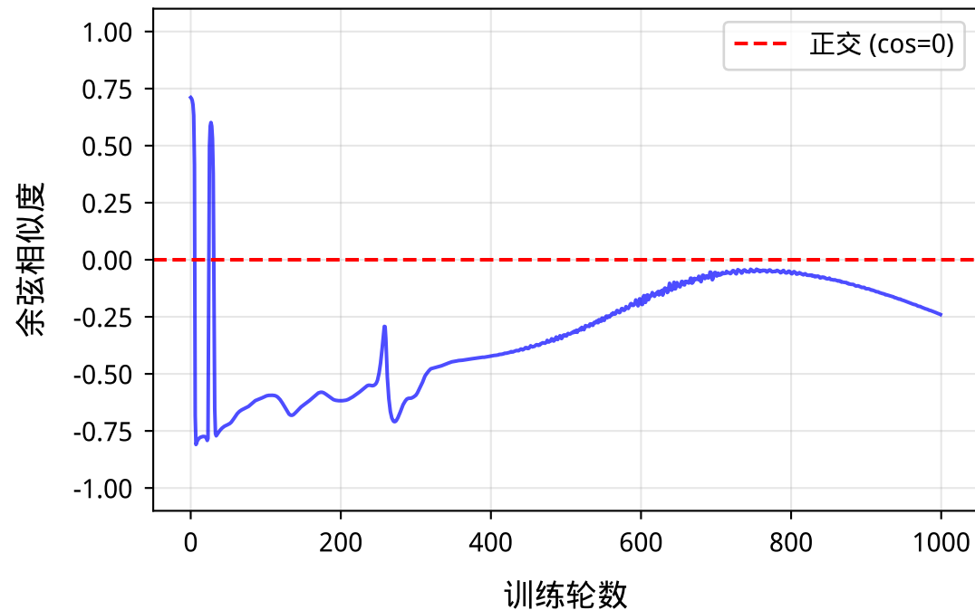
PDE梯度与边界条件梯度的夹角
