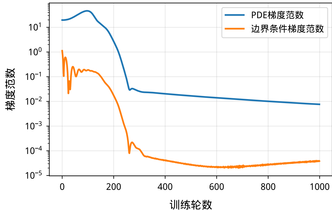
各项损失的梯度范数
