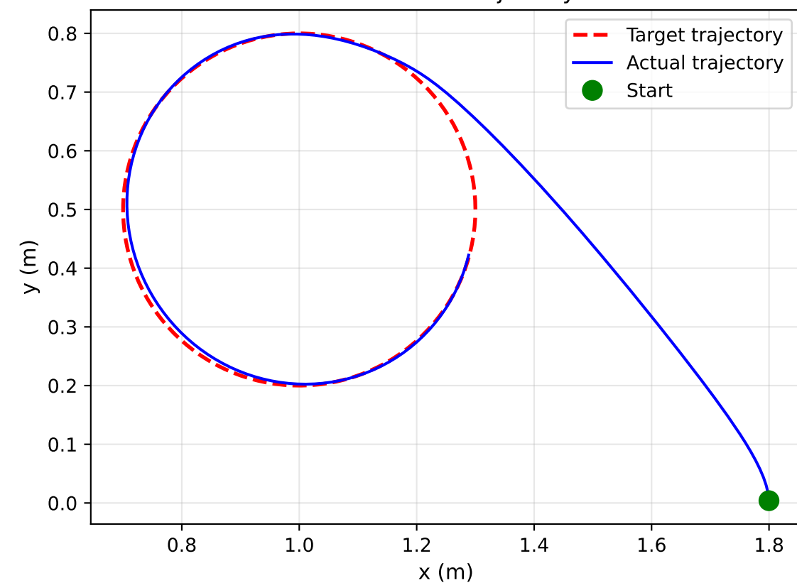
End-effector Trajectory
