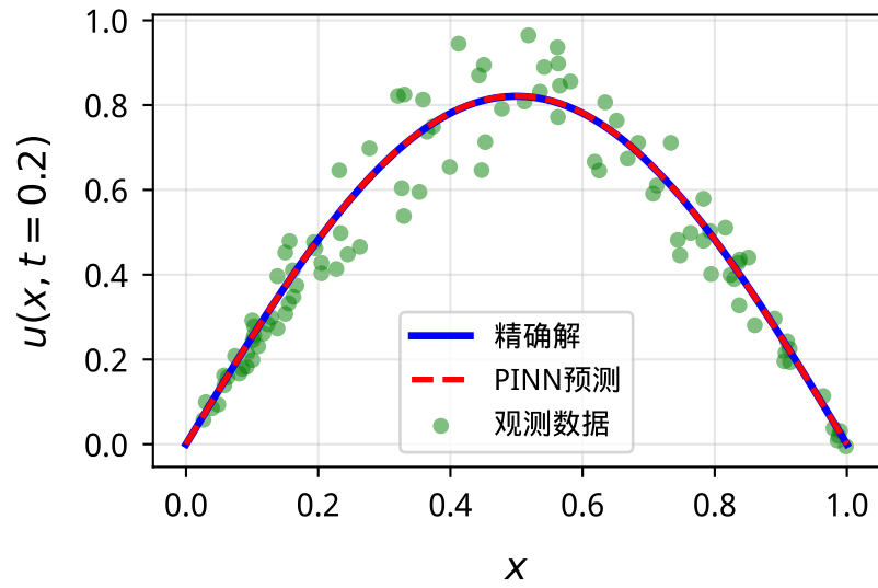
t = 0.2 时刻解对比 (反演 D=0.0995 , 真实 D=0.1 )
