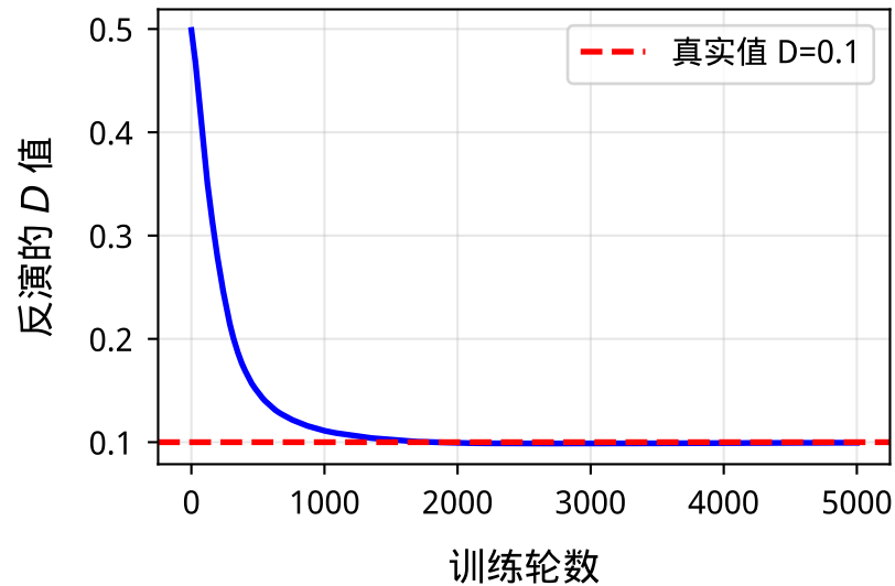
扩散系数反演过程
