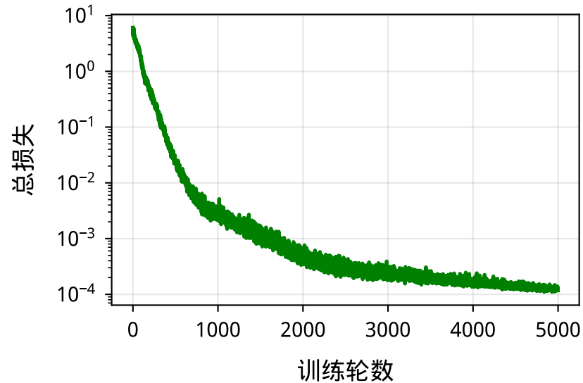
训练损失曲线
