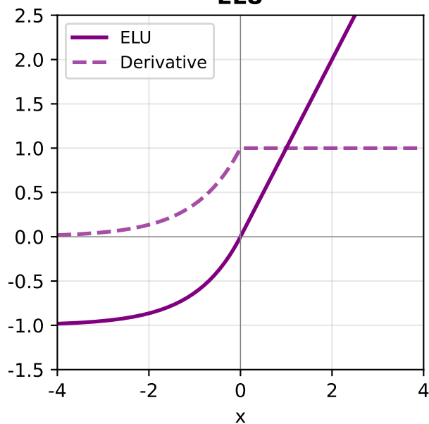
ELU
