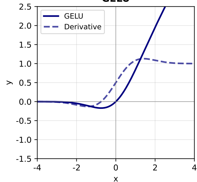
GELU
