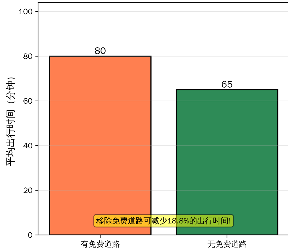
Braess悖论: 增加免费道路反而更慢!
