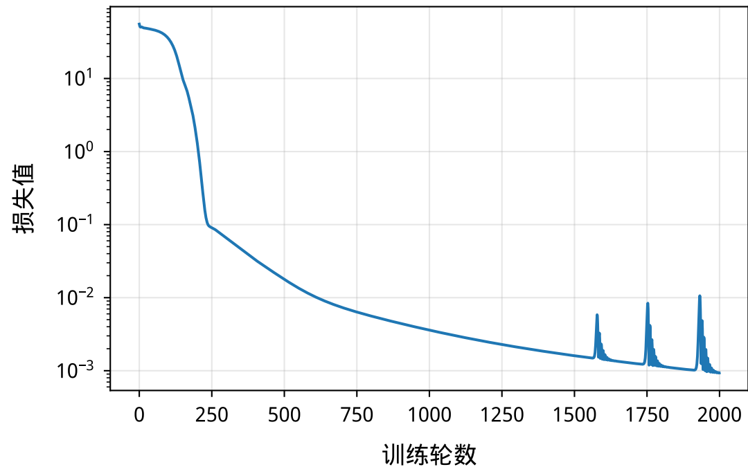
训练损失曲线
