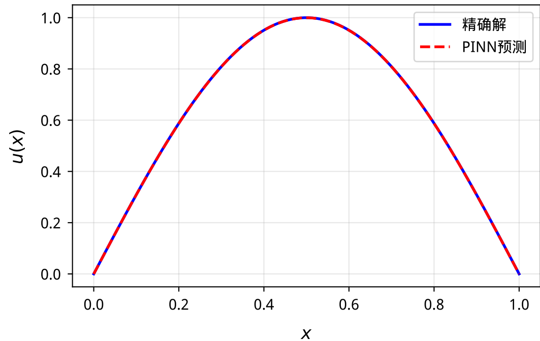
PINN解与精确解对比
