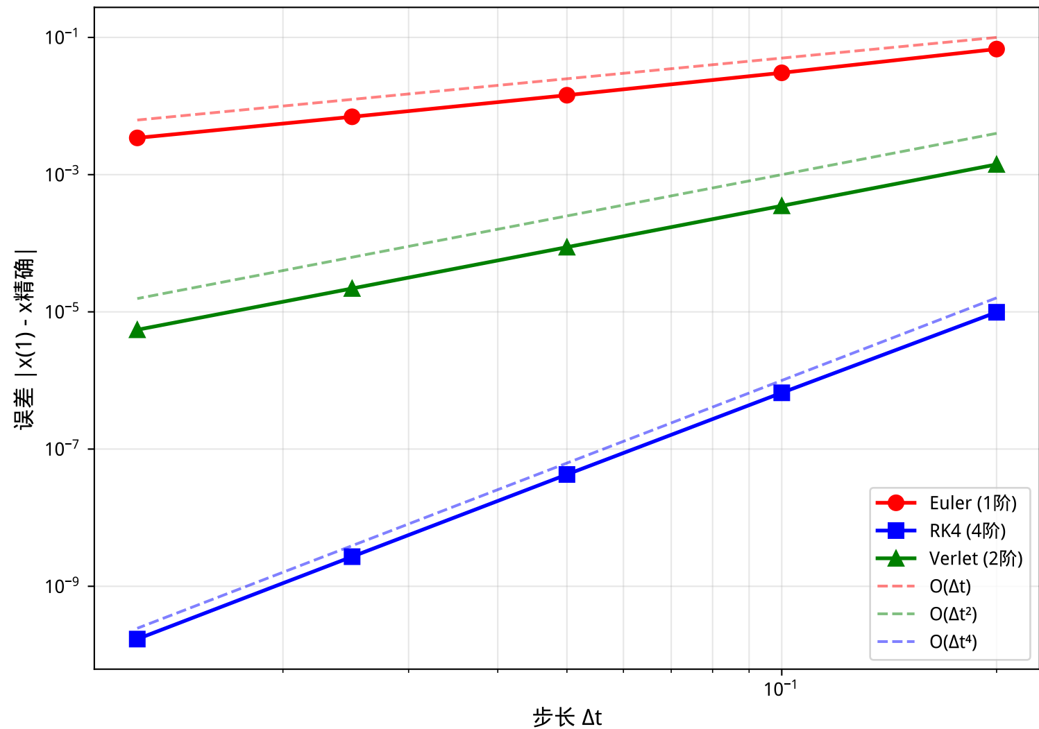
收敛阶验证
