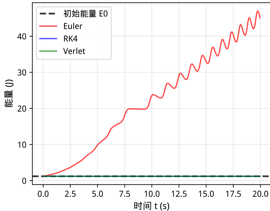
能量守恒对比
