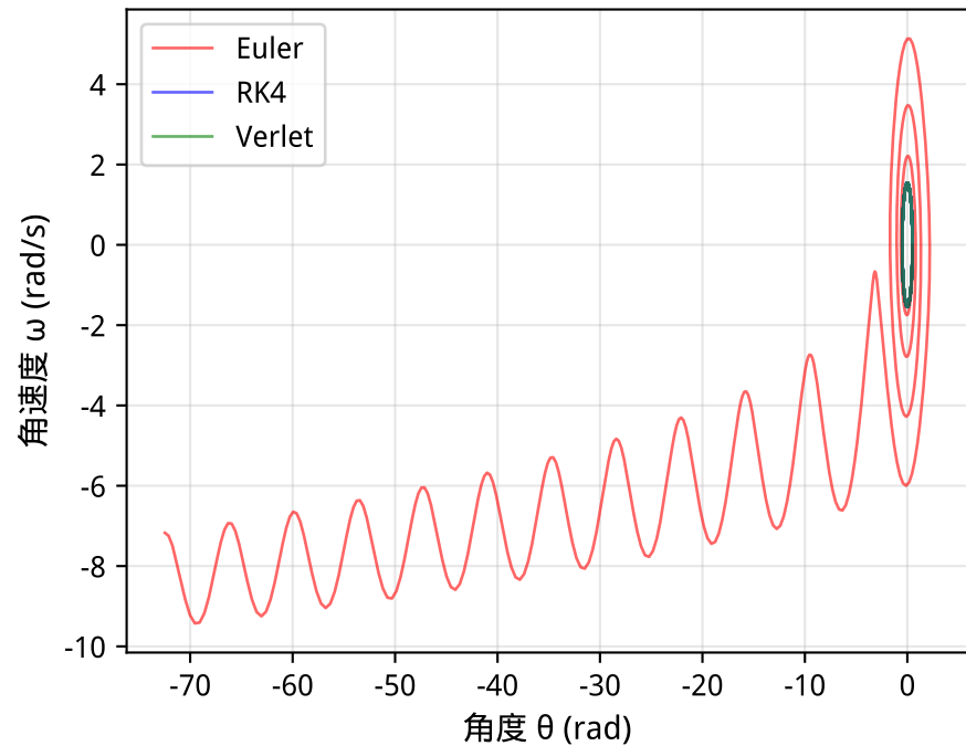
相空间轨迹
