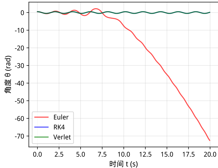
单摆：角度随时间变化
