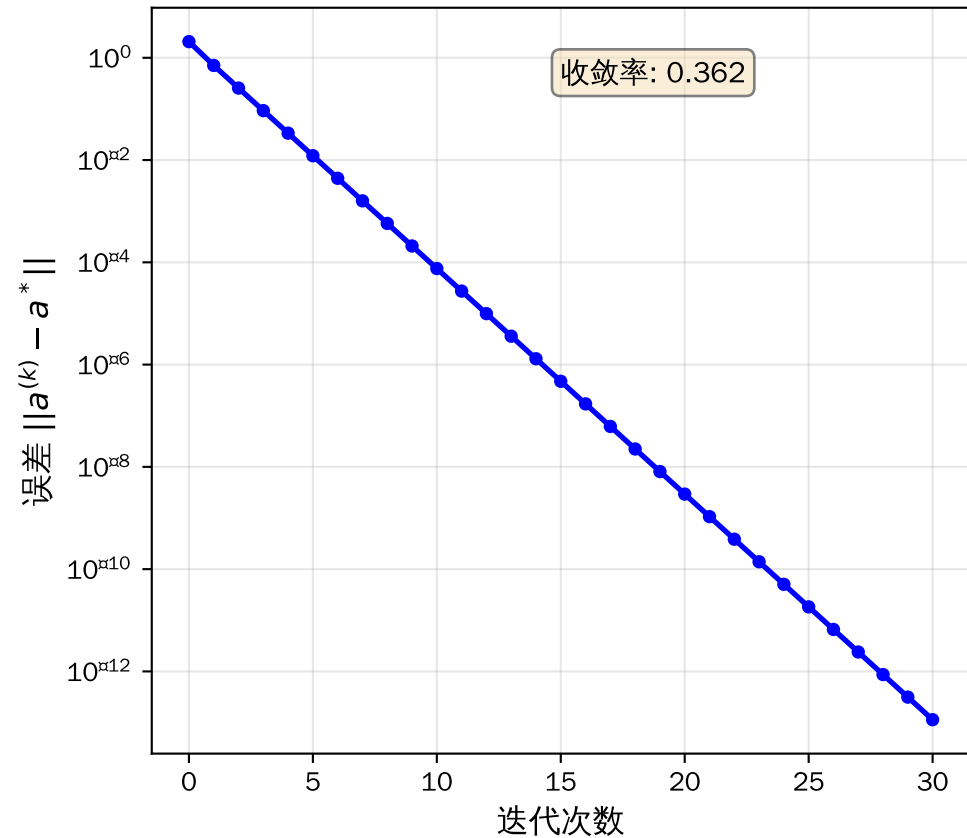
收敛速率 (线性收敛)
