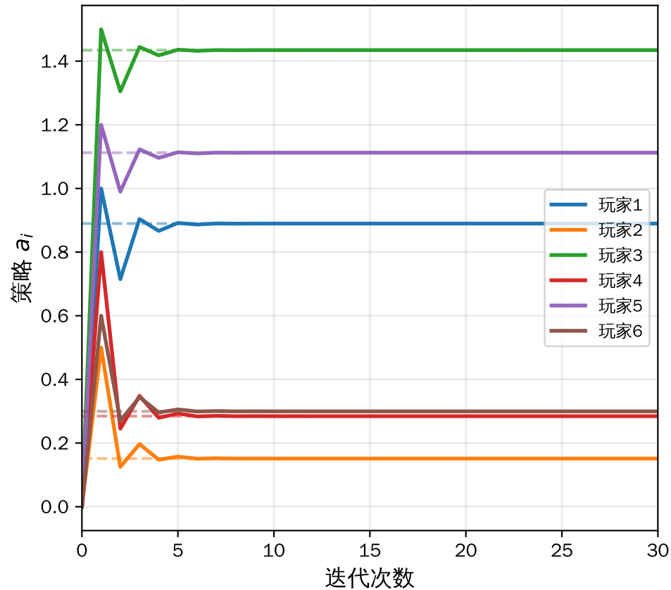
迭代最优响应收敛过程 (虚线=纳什均衡)
