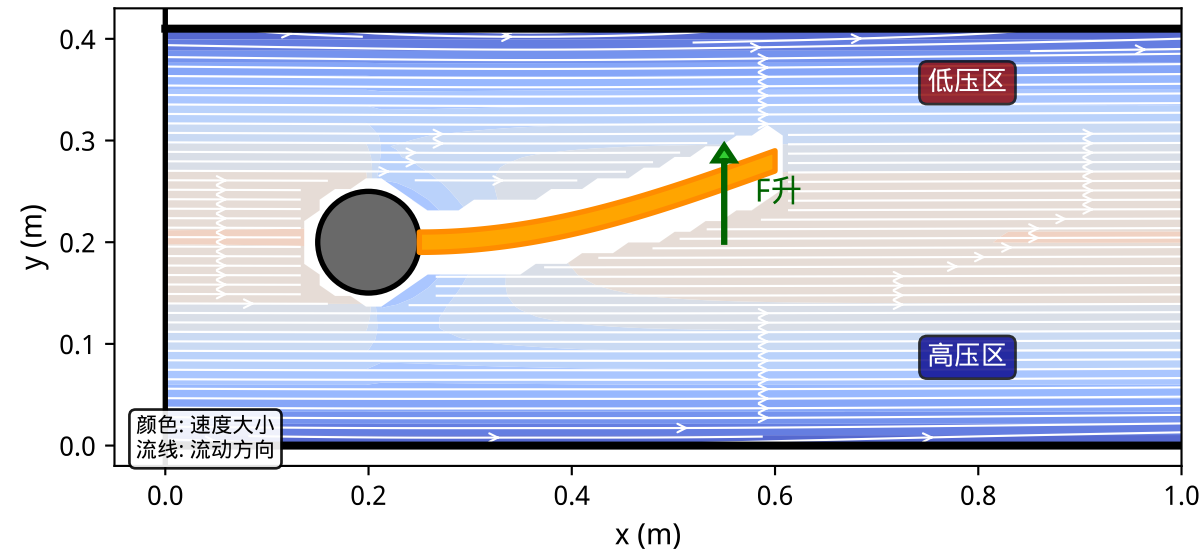
(a) 板向上运动：上方涡脱落
