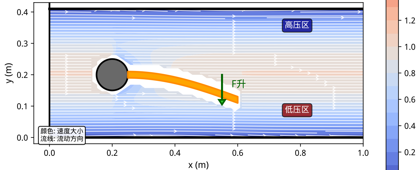
(b) 板向下运动：下方涡脱落
