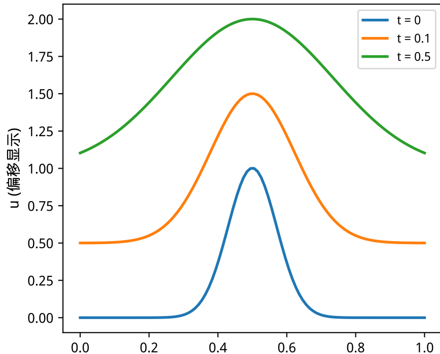
抛物型: 热方程
