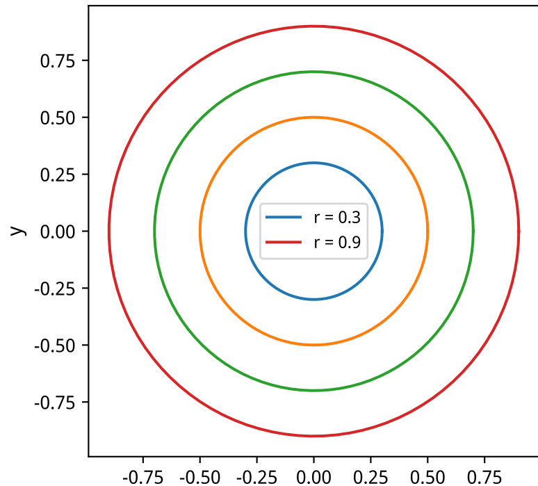
椭圆型: Laplace方程
