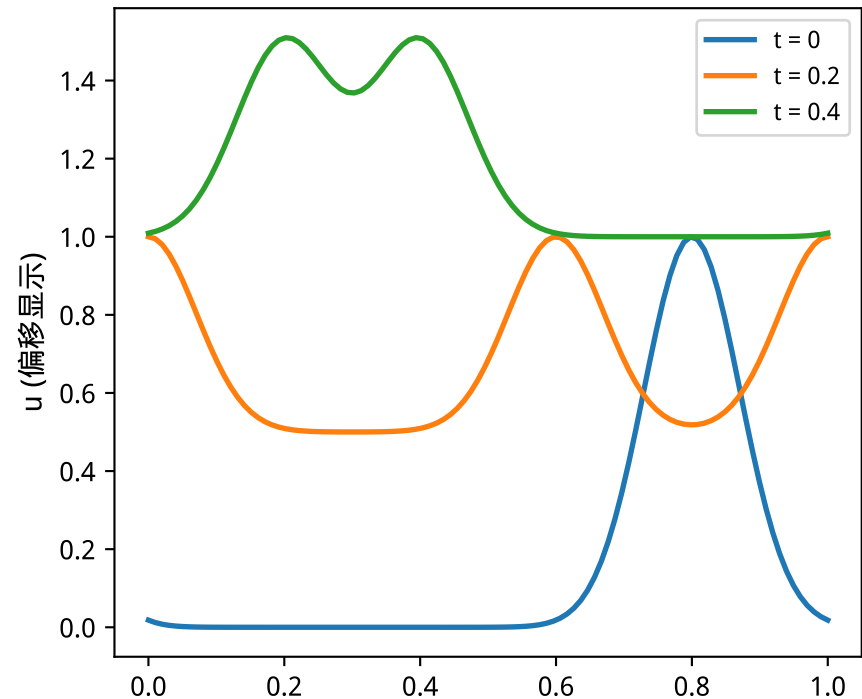
双曲型: 波动方程
