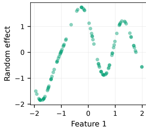
Task 7
