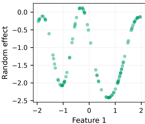
Task 5
