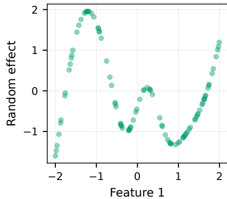
Task 5
