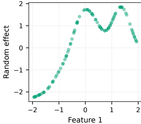
Task 6
