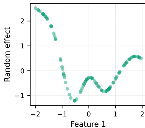
Task 7
