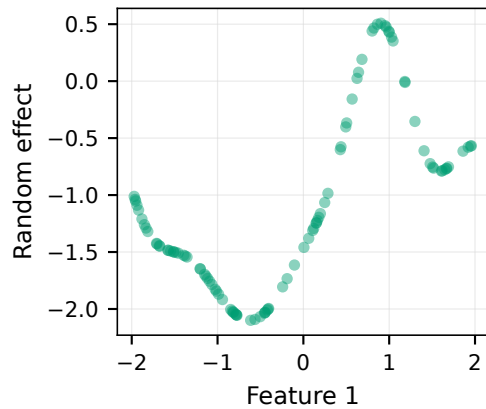
Task 8
