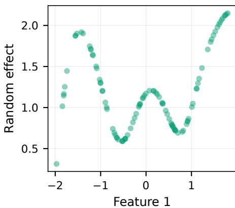
Task 6
