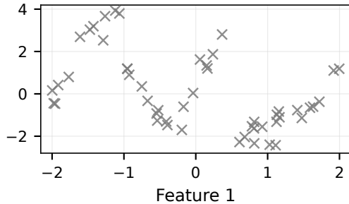
Task 1
