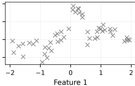
Task 2
