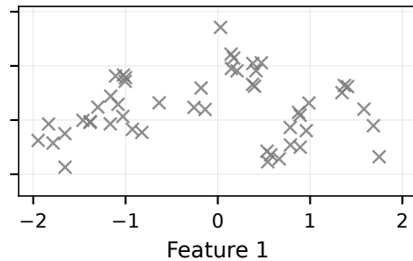
Task 3
