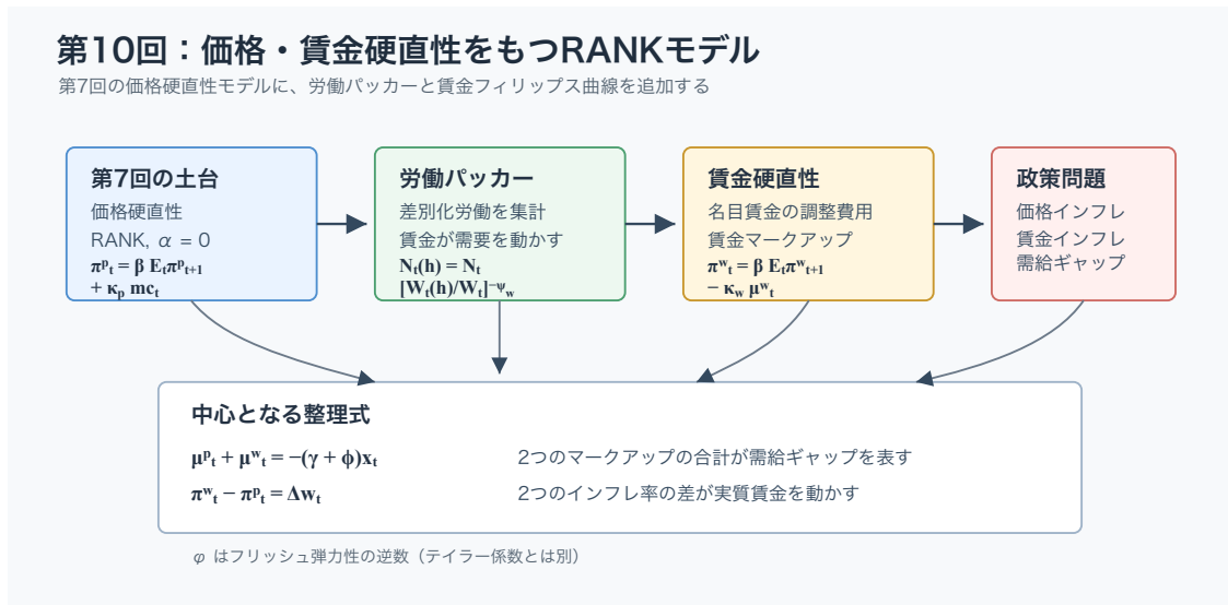
図1: 第10回講義の全体像:第7回の価格硬直性RANKモデルに労働パッカーと賃金調整費用を加えると、 \mu_t^p + \mu_t^w = -(\gamma + \phi)x_t と \pi_t^w - \pi_t^p = \Delta w_t が価格・賃金ブロックを結ぶ。
