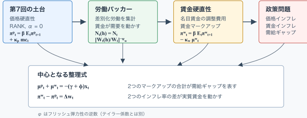
図 1: 第 10 回講義の全体像：第 7 回の価格硬直性 RANK モデルに労働パッカーと賃金調整費用を加えると、 \mu_t^p + \mu_t^w = -(\gamma + \phi)x_t と \pi_t^w - \pi_t^p = \Delta w_t が価格・賃金ブロックを結ぶ。
