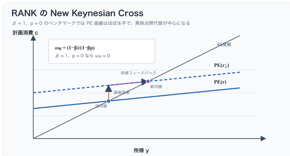
図 2: RANK の NK クロス ( \beta = 0.99 、 p = 0 )。この較正では PE 曲線はほぼ水平で、実質利子率ギャップの低下は主に直接シフトとして現れる。一般に「ほぼ水平」には \beta \simeq 1 に加えて p が 1 に近すぎないことが必要である。
