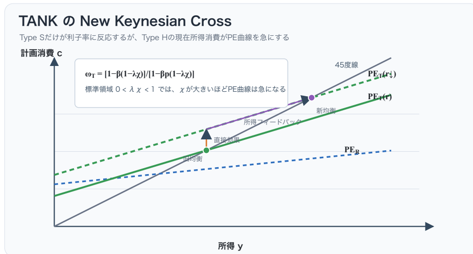
図 4: TANK の NK クロス。実質利子率ギャップに直接反応するのは Type S だけなので直接シフトは小さいが、Type H の現在所得消費により PE 曲線の傾きは大きくなる。
