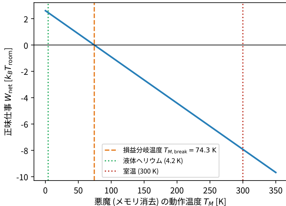
(b) メモリ温度に対する正味仕事と損益分岐点
