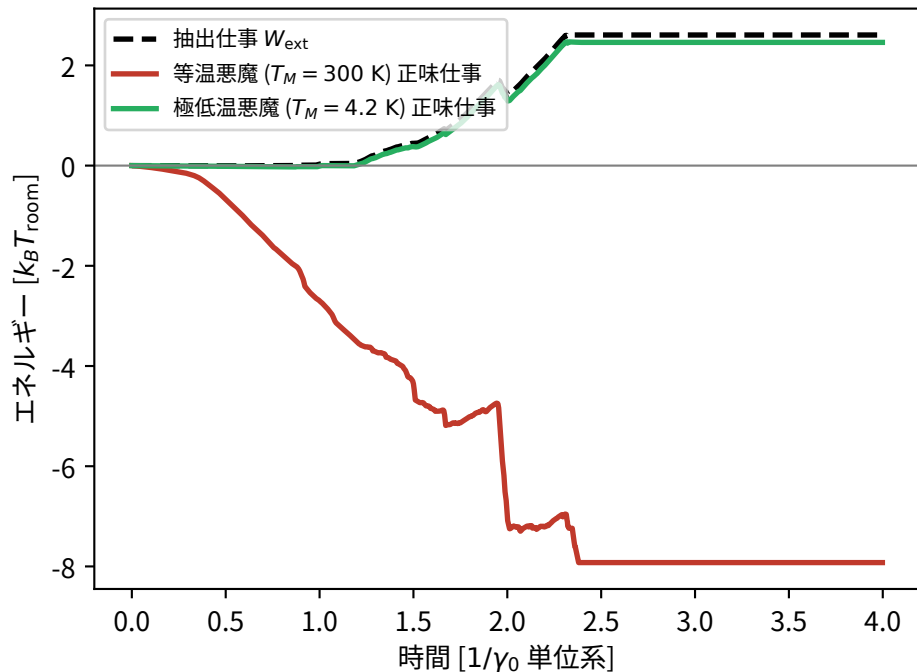
(a) 時間発展と消去コスト
