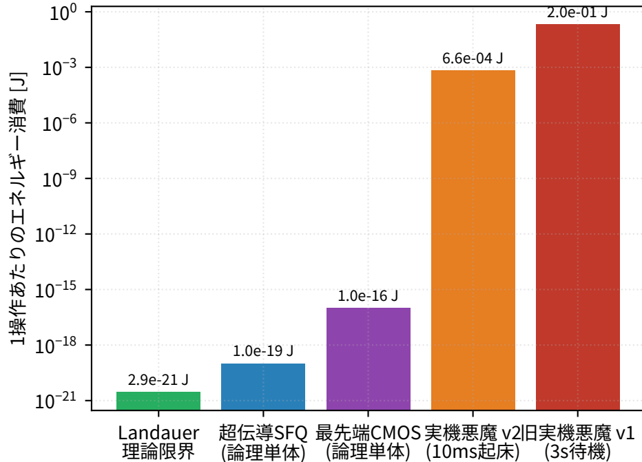
(a) 理論限界と現実の悪魔の17桁のギャップ
