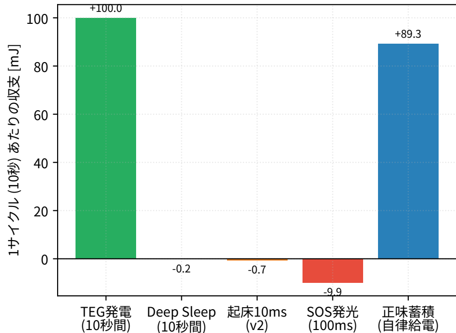
(b) 構成D実機における自律給電エネルギー収支 ( \Delta T=15^\circ\text{C} )
