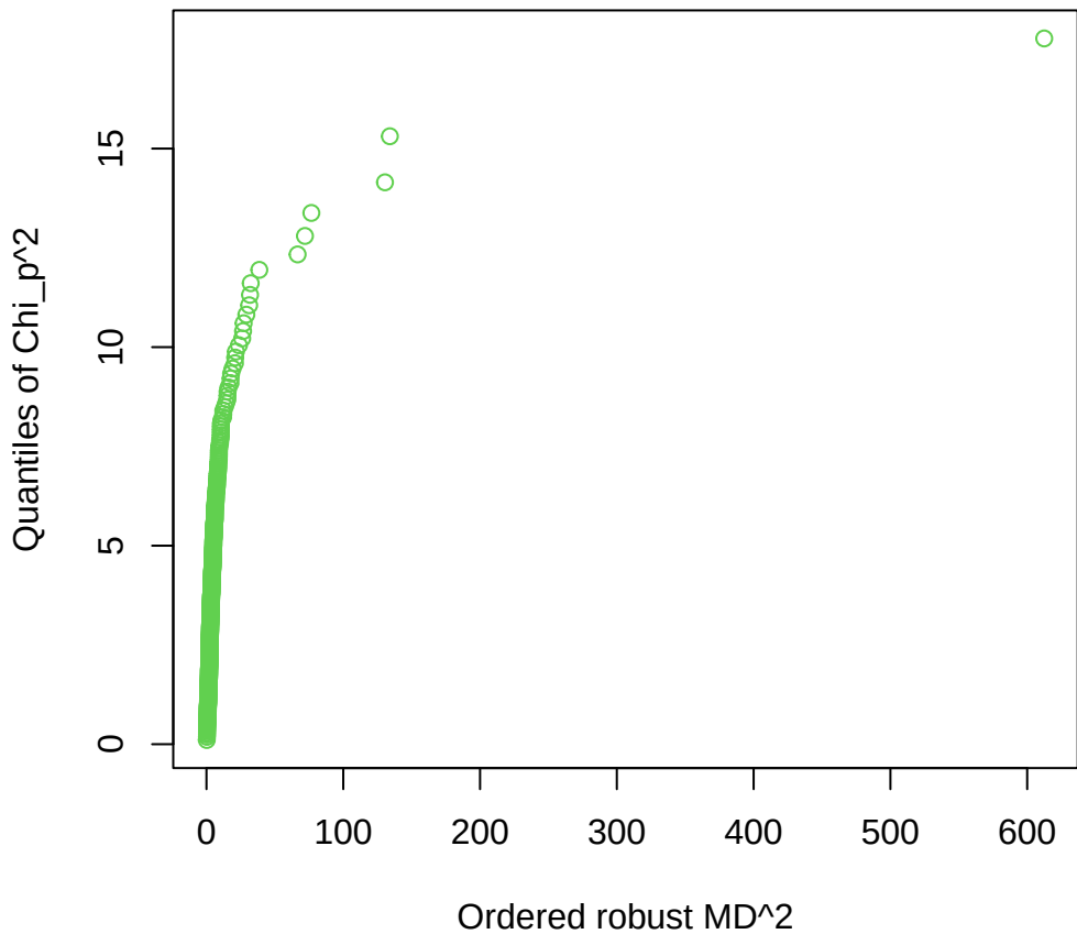
Chi 2 -Plot
