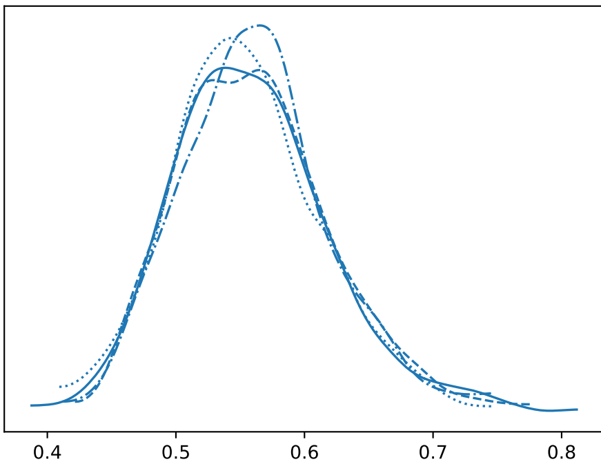
tau2
