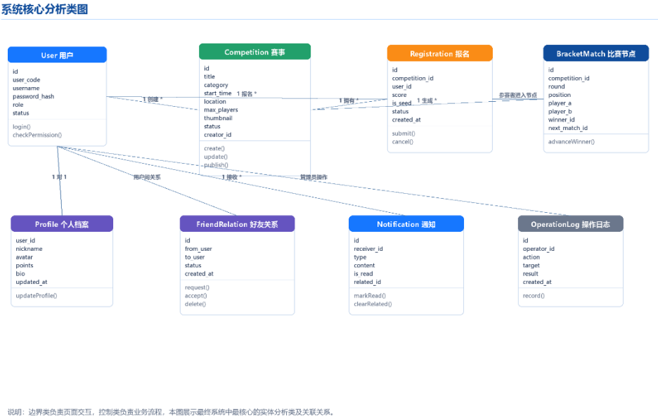
图 3-12 系统核心分析类图
