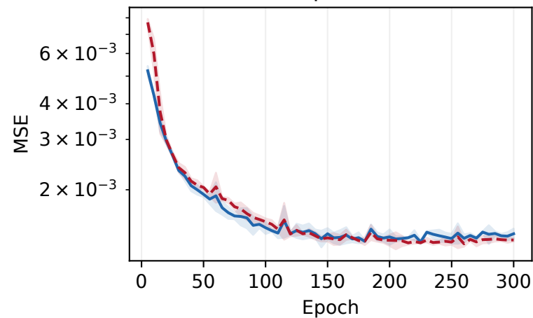
dSprites
