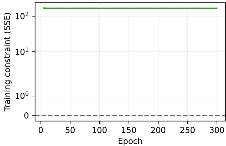
dSprites
