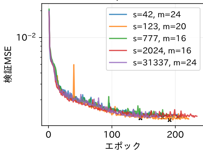
dSprites
