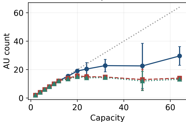
dSprites
