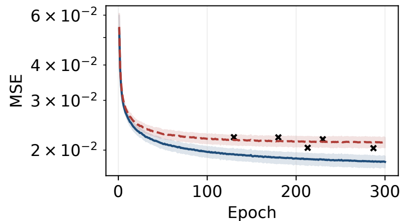
MNIST, m=32
