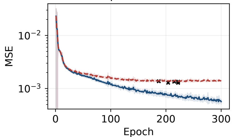
dSprites, m=32
