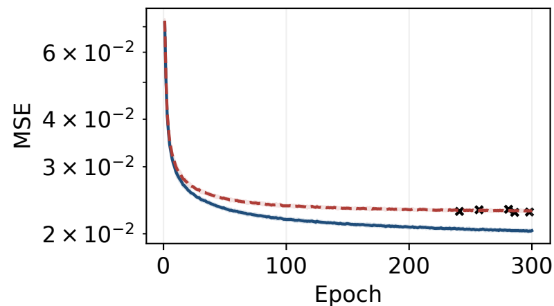
MNIST, m=64
