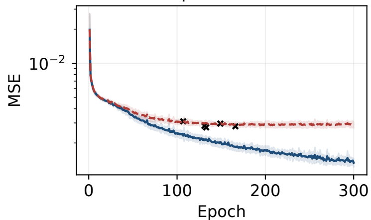
dSprites, m=16
