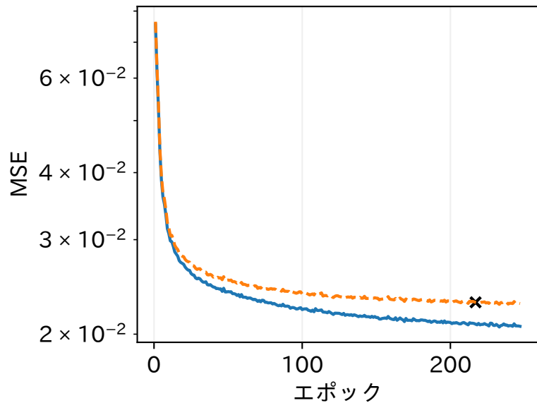
MNIST, 64次元
