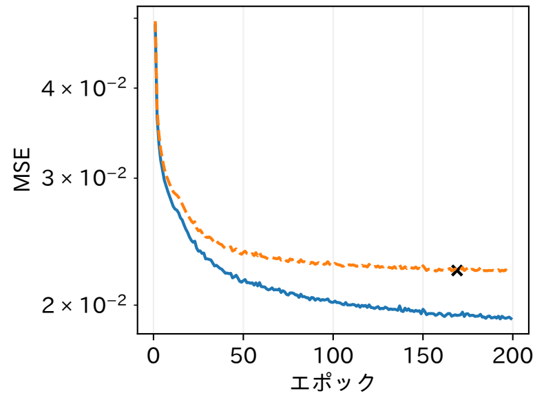
MNIST, 6次元
