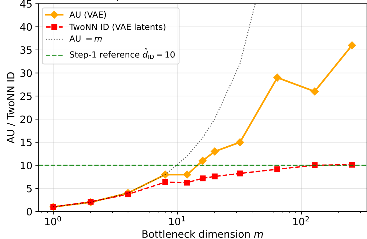
(d) VAE ( \beta = 4 ): AU and latent TwoNN ID vs. m
