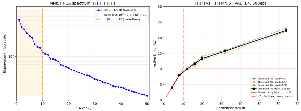
図 2: 実験 EM: (左) MNIST PCA 固有値スペクトルと線形理論の水充填水面 ( \beta\tau^2 \approx 1.18 , d^* = 10 ). (右) 線形理論の予測 (赤実線; d^* = 10 で鋭い飽和を仮定) と非線形 FC-VAE の観測 AU(m) 曲線 (各シード・平均) の比較. 非線形 VAE での AU 増加は緩やかであり, m^{\text{knee}} の不安定性の理論的根拠を示す.
