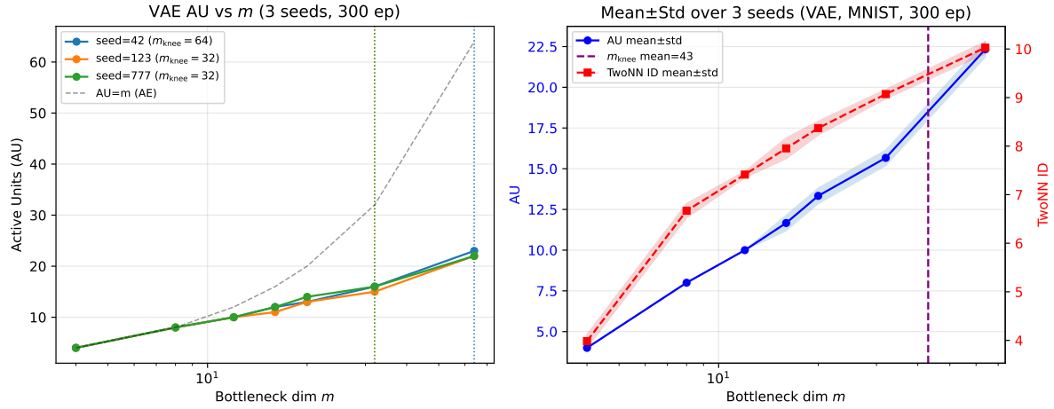
図 4: E4-300ep-multiseed : MNIST VAE の AU パターン (3 シード, 300 エポック). 左: 各シードの AU vs m (点線は m^{\text{knee}} ); 右: 平均 \pm 標準偏差バンド. AU \cdot TwoNN ID のバンドは非常に狭いが, m^{\text{knee}} はシード間で 32~64 に変動する.
