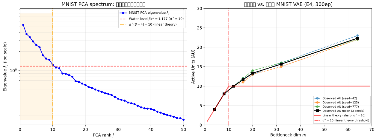
図 5: 実験 EM：(左) MNIST PCA 固有値スペクトルと線形理論の水充填水面 ( \beta\tau^2 \approx 1.18 , d^* = 10 ). (右) 線形理論の予測（赤実線； d^* = 10 で鋭い飽和を仮定）と非線形 FC-VAE の観測 AU( m ) 曲線（各シード・平均）の比較. 非線形 VAE での AU 増加は緩やかであり、 m^{\text{knee}} の不安定性の理論的根拠を示す.
