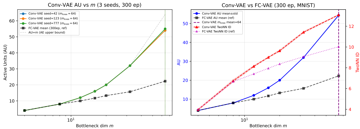
図 9: EH: Conv-VAE 300ep の AU パターンと FC-VAE との比較. 左: 各シードの AU vs m (点線は m^{\text{knee}}=64 ); 右: Conv-VAE と FC-VAE の平均 \pm 標準偏差バンド比較. Conv-VAE は m \leq 32 で AU = m (KL 飽和なし) であり, FC-VAE との顕著な差を示す.
