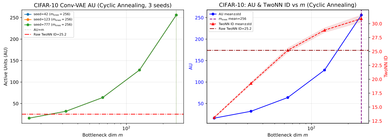
図 12: EI: CIFAR-10 Conv-VAE (KL サイクリックアニーリング) における AU・TwoNN ID の m 依存性 (3 シード). TwoNN ID は Pope ら [17] の報告値 ( d_{\text{ID}} \approx 26 ) と収束傾向を示す.
