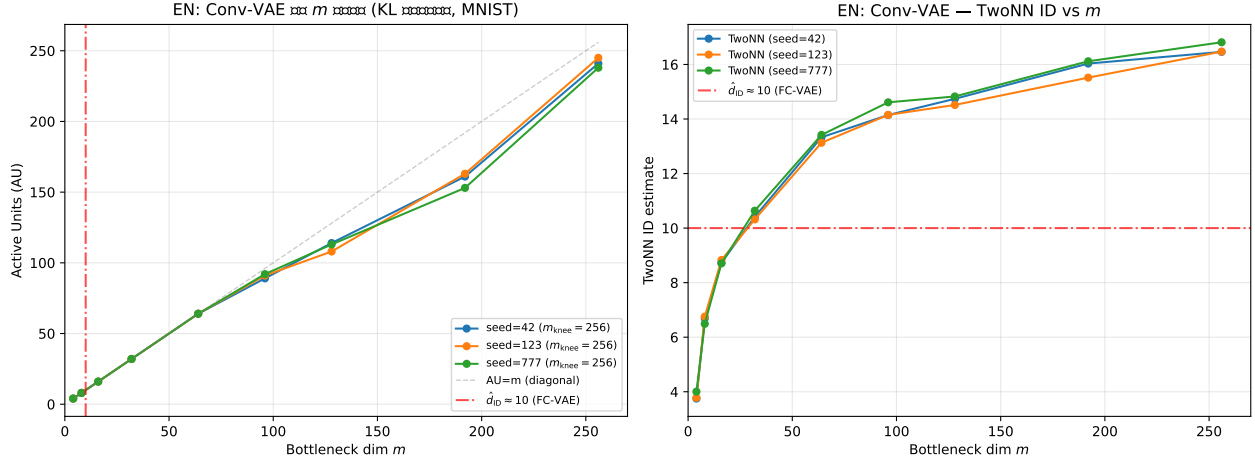
図 11: 実験 EN: Conv-VAE 拡張 m グリッド ( m \in [4, 256] , KL アニール, 3 シード) の AU vs m (左) および TwoNN ID vs m (右). 対角線 ( AU=m ) と FC-VAE の \hat{d}_{\text{ID}} \approx 10 参照線 (赤) を示す. m \leq 64 では AU=m (対角線上) が続くが, m \geq 96 で対角線から離れ始め, Conv-VAE でも水充填原理の定性的傾向が確認できる.
