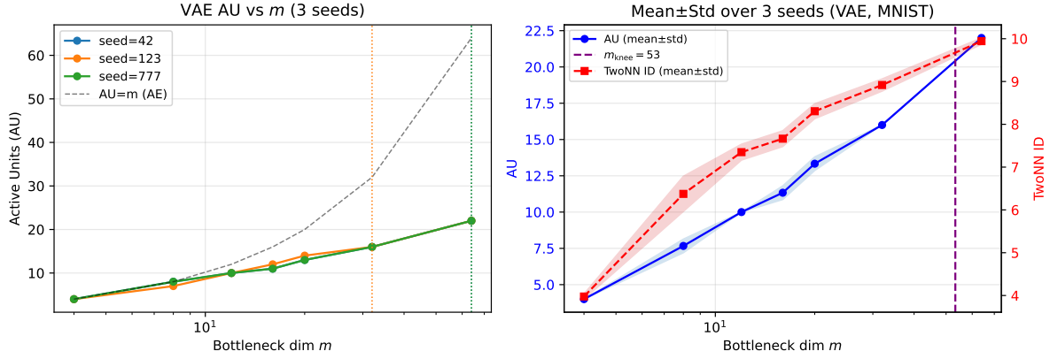
図 3: E4-multiseed : MNIST VAE の AU パターン (3 シード). 左: 各シードの AU vs m (点線は各シードの m^{\text{knee}} ) ; 右: 平均 ± 標準偏差バンド. AU 値はシード間で高度に一致するが, m^{\text{knee}} は 32~64 に変動する.
