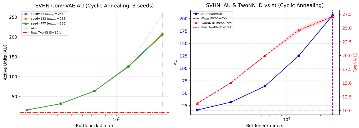
図 13: EJ: SVHN Conv-VAE (KL サイクリックアニーリング) における AU・TwoNN ID の m 依存性 (3 シード).
