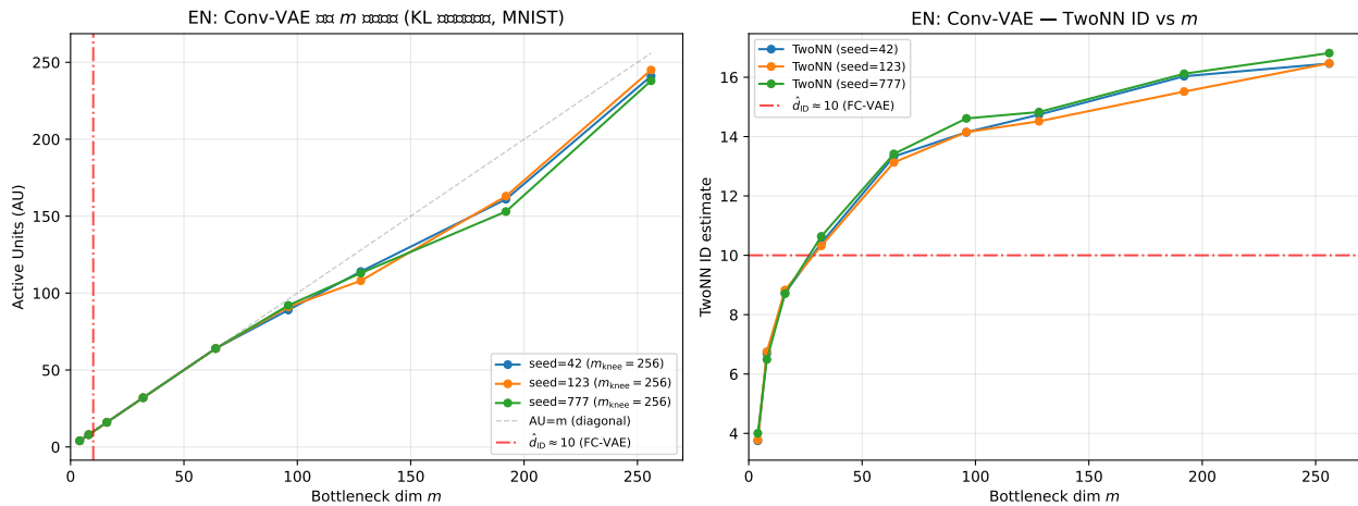
図 12: 実験 EN : Conv-VAE 拡張 m グリッド ( m \in [4, 256] , KL アニールリング, 3 シード) の AU vs m (左) および TwoNN ID vs m (右). 対角線 ( AU = m ) と FC-VAE の \hat{d}_{ID} \approx 10 参照線 (赤) を示す. m \leq 64 では AU = m (対角線上) が続くが, m \geq 96 で対角線から離れ始め, Conv-VAE でも水充填原理の定性的傾向が確認できる.
