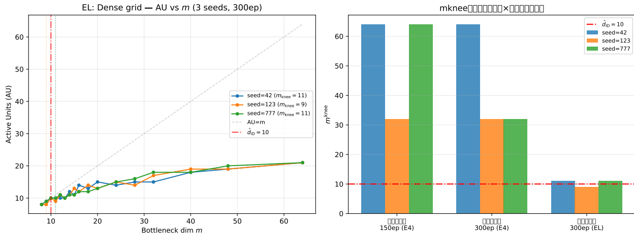
図 7: EL：(左) 密グリッドの AU vs m (3 シード). (右) グリッド密度 \times エポックの比較. 密グリッドでの m^{\text{knee}} 変動は命題 2 の上界 (最大グリッド間隔) で評価できる.
