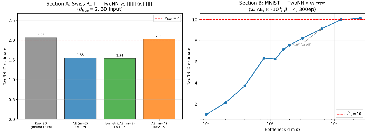
図 2: 実験 EP: (左) Swiss Roll での TwoNN ID 棒グラフ— m = d_{\text{true}} = 2 では AE・IsometricAE とともに TwoNN \approx 1.55 と過小推定 ( \kappa の差よりボトルネック余裕の不足が主因); m = 4 > d_{\text{true}} で TwoNN が 2.03 へ回復. (右) MNIST での TwoNN vs m 収束曲線 (参照 AE, \kappa \approx 10^9 ): m \geq 128 で TwoNN が \approx 10 に収束し, m \gg d_{\text{ID}} 条件下での数値的安定性を示す.
