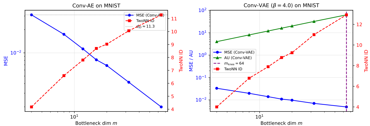
図 9: EG : Conv-AE (左) \cdot Conv-VAE (右) における MSE, AU, TwoNN ID の m 依存性 (MNIST, 100 エポック). Conv-AE では AU = m (全次元活性) が確認され、TwoNN ID が m \geq 32 で \approx 11 に収束する。Conv-VAE では AU \approx m (100 エポックの収束不足により飽和なし)。
