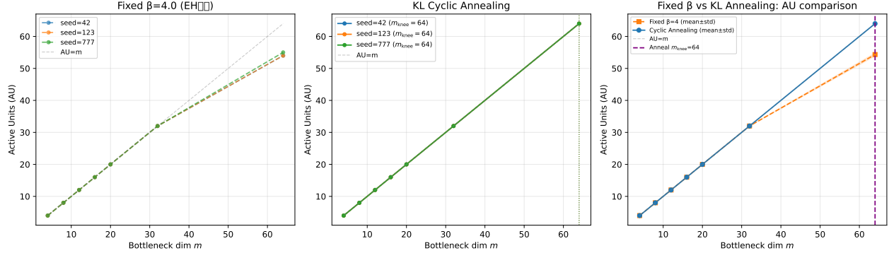
図 11: EK：固定 \beta (左) vs KL サイクリックアニーリング (中央) の各シード AU 曲線，および平均比較 (右)．固定 \beta では m = 64 のみで部分的崩壊 ( AU \approx 54 ) が生じるが，アニーリングでは全次元が常に活性 ( AU = m ) となり， m \in [4, 64] の範囲ではいずれの条件でも明確な AU 飽和 ( AU が m を下回るプラトー) は観測されなかった。
