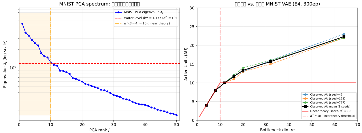
図 6: 実験 EM：(左) MNIST PCA 固有値スペクトルと線形理論の水充填水面 ( \beta\tau^2 \approx 1.18 , d^* = 10 ). (右) 線形理論の予測（赤実線； d^* = 10 で鋭い飽和を仮定）と非線形 FC-VAE の観測 AU( m ) 曲線（各シード・平均）の比較. 非線形 VAE での AU 増加は緩やかであり、 m^{\text{knee}} の不安定性の理論的根拠を示す.
