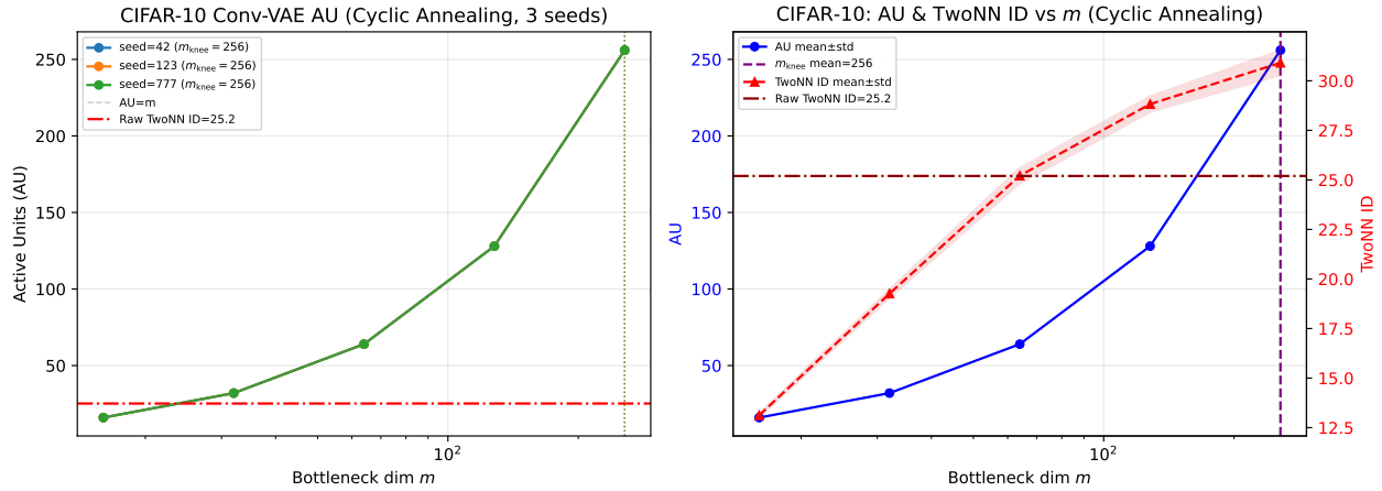
図 13: EI: CIFAR-10 Conv-VAE (KL サイクリックアニーリング) における AU・TwoNN ID の m 依存性 (3 シード). TwoNN ID は Pope ら [17] の報告値 ( d_{\text{ID}} \approx 26 ) と収束傾向を示す.
