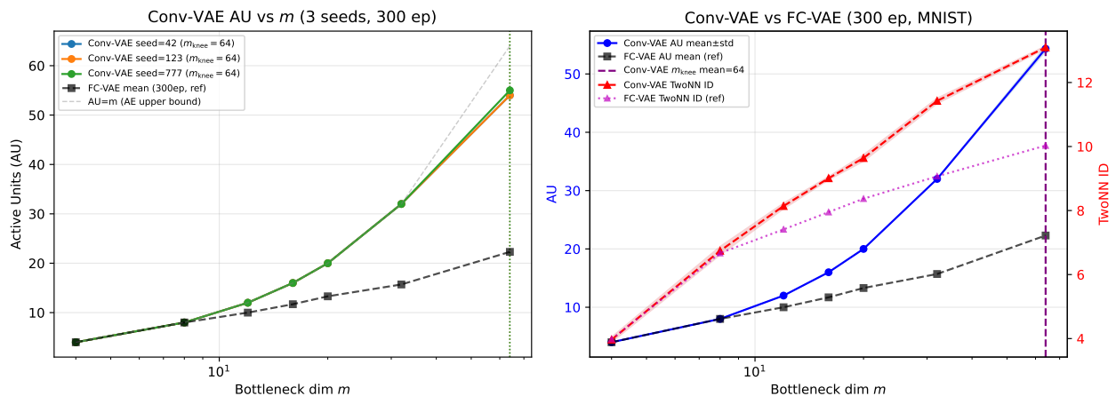
図 10: EH : Conv-VAE 300ep の AU パターンと FC-VAE との比較. 左: 各シードの AU vs m (点線は m^{\text{knee}}=64 ); 右: Conv-VAE と FC-VAE の平均 \pm 標準偏差バンド比較. Conv-VAE は m \leq 32 で AU = m (KL 飽和なし) であり, FC-VAE との顕著な差を示す.
