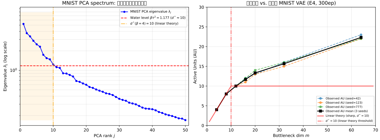
図 6: 実験 EM: (左) MNIST PCA 固有値スペクトルと線形理論の水充填水面 ( \beta\tau^2 \approx 1.18 , d^* = 10 ). (右) 線形理論の予測 (赤実線; d^* = 10 で鋭い飽和を仮定) と非線形 FC-VAE の観測 AU(m) 曲線 (各シード・平均) の比較. 非線形 VAE での AU 増加は緩やかであり, m^{\text{knee}} の不安定性の理論的根拠を示す.
