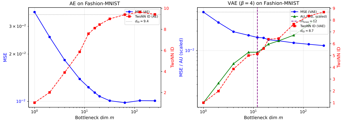
図 8: EF : Fashion-MNIST の AE (左)・VAE (右) における MSE, AU, TwoNN ID の m 依存性 (100 エポック). VAE では m = 12 付近 ( \tau_{\text{knee}} = 0.25 での m^{\text{knee}} ) で AU 成長率が急減し, TwoNN ID は m \geq 32 で \approx 9.4 (AE)・ \approx 8.7 (VAE) に漸近的に収束する.
