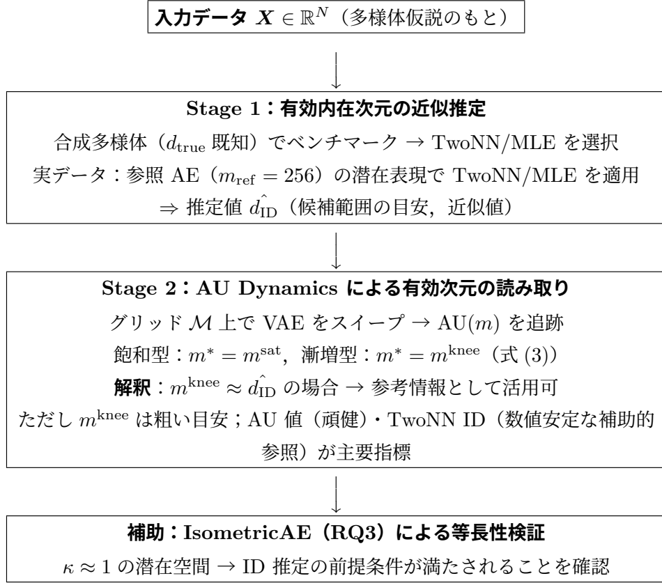
図 1: 有効潜在次元の読み取りパイプライン. m^{\text{knee}} は設計目安であると同時に, 「VAE が実際に何次元の有効表現を学習するか」を外部から読む解釈指標である.
