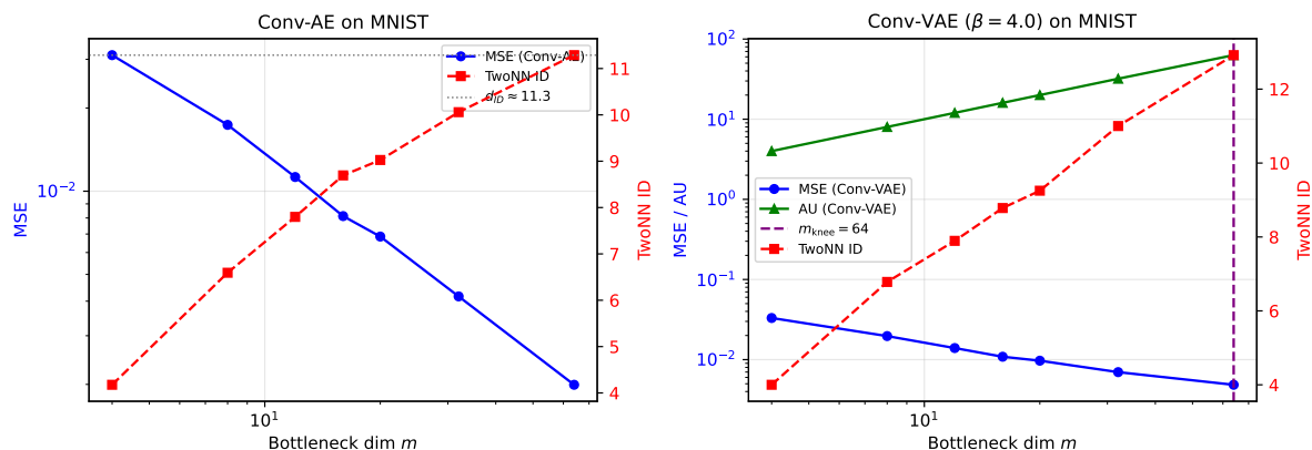
図 9: EG：Conv-AE (左)・Conv-VAE (右) における MSE, AU, TwoNN ID の m 依存性 (MNIST, 100 エポック). Conv-AE では AU = m (全次元活性) が確認され, TwoNN ID が m \geq 32 で \approx 11 に収束する. Conv-VAE では AU \approx m (100 エポックの収束不足により飽和なし).
