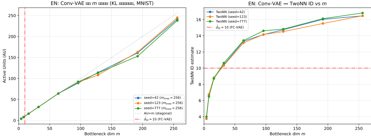
図 10: 実験 Exp-Conv-M256 : Conv-VAE 拡張 m グリッド ( m \in [4, 256] , KL アニールグ, 3 シード) の AU vs m (左) および TwoNN ID vs m (右). 対角線 ( AU = m ) と FC-VAE の \hat{d}_{ID} \approx 10 参照線 (赤) を示す. m \leq 64 では AU = m (対角線上) が続くが, m \geq 96 で対角線から離れ始め, Conv-VAE でも水充填原理の定性的傾向が確認できる.
