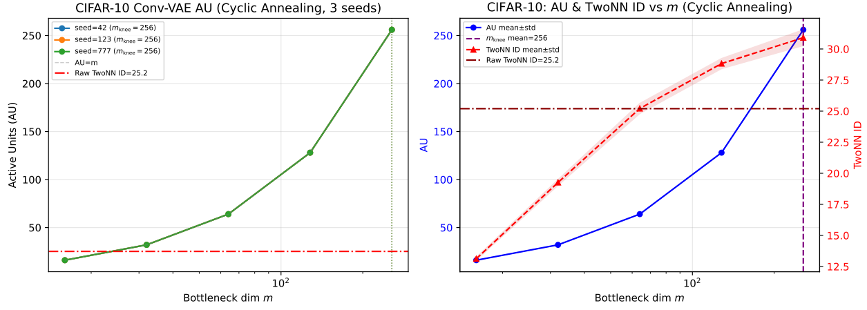
図 12: Exp-Nat-Cifar : CIFAR-10 Conv-VAE (KL サイクリックアニーリング) における AU・TwoNN ID の m 依存性 (3 シード). TwoNN ID は Pope ら [17] の報告値 ( d_{ID} \approx 26 ) と収束傾向を示す.
