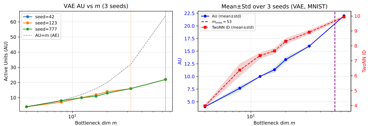
図 4: Exp-Mnist-Multi : MNIST VAE の AU パターン (3 シード). 左: 各シードの AU vs m (点線は各シードの m^{\text{knee}} ); 右: 平均 \pm 標準偏差バンド. AU 値はシード間で高度に一致するが, m^{\text{knee}} は 32~64 に変動する.
