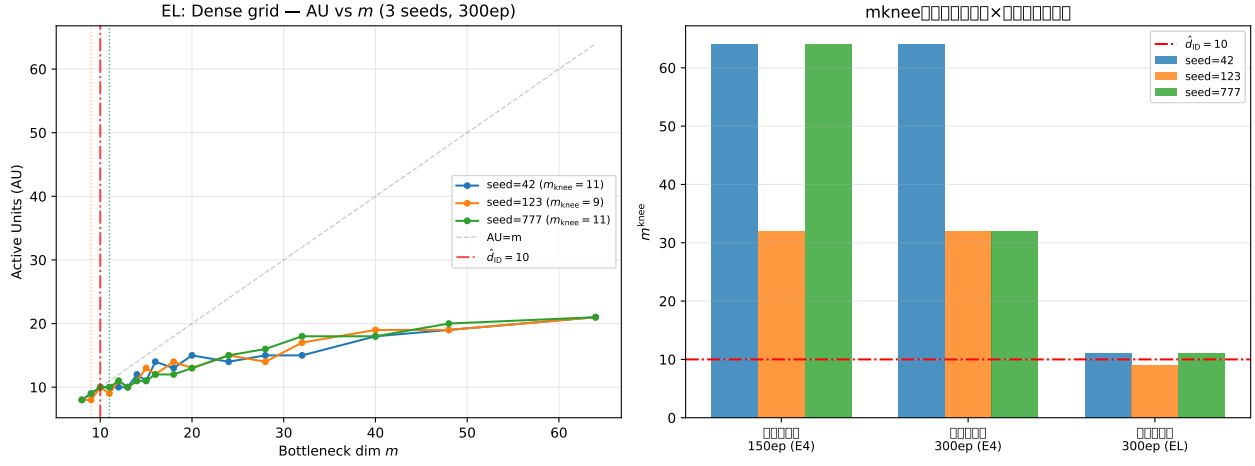
図 7: Exp-Mnist-Dense : (左) 密グリッドの AU vs m (3 シード). (右) グリッド密度×エポックの比較. 密グリッドでの m^{\text{knee}} 変動は命題 2 の上界 (最大グリッド間隔) で評価できる.
