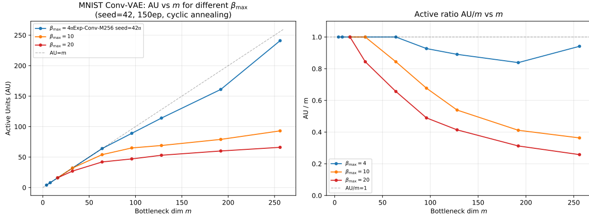
図 11: Exp-ConvV-HiBeta : \beta_{\max} \in \{4, 10, 20\} での MNIST Conv-VAE AU vs m (左) および活性率 AU/m (右) の比較. \beta_{\max} を増大させると AU 飽和が低次元側に現れ, d^*(\beta) の \beta 依存性を実証する.
