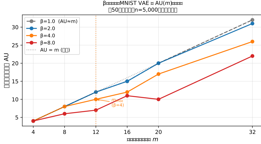
図 14: \beta 感度分析：MNIST VAE の AU vs m ( \beta \in \{1, 2, 4, 8\} , 50 エポック, サブセット). \beta = 1 では AU \approx m (正則化不足), \beta = 4 では m_{\text{knee}} = 12 (垂直破線), \beta = 8 では m < 8 で AU が過度に抑制される兆候が見られる.
