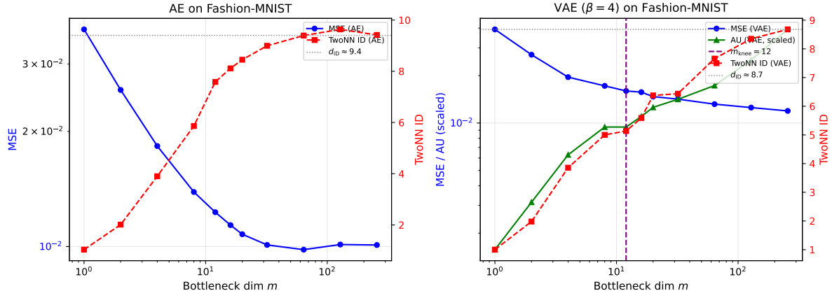
図 8: Exp-Fashion : Fashion-MNIST の AE (左)・VAE (右) における MSE, AU, TwoNN ID の m 依存性 (100 エポック). VAE では m = 12 付近 ( \tau_{\text{knee}} = 0.25 での m^{\text{knee}} ) で AU 成長率が急減し, TwoNN ID は m \geq 32 で \approx 9.4 (AE)・ \approx 8.7 (VAE) に漸的に収束する.
