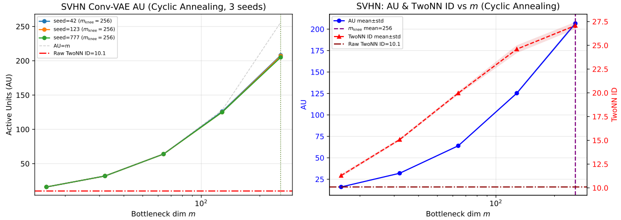
図 13: Exp-Nat-SVHN : SVHN Conv-VAE (KL サイクリックアニーリング) における AU・TwoNN ID の m 依存性 (3 シード).
