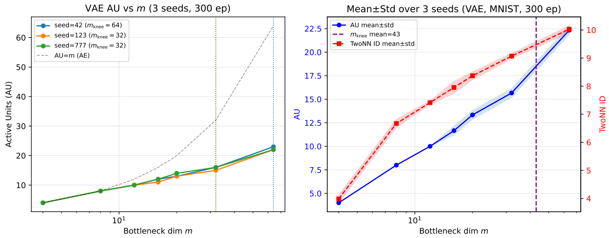
図 5: Exp-Mnist-Multi : MNIST VAE の AU パターン (3 シード, 300 エポック). 左: 各シードの AU vs m (点線は m^{\text{knee}} ); 右: 平均 ± 標準偏差バンド. AU・TwoNN ID のバンドは非常に狭いが, m^{\text{knee}} はシード間で 32~64 に変動する.
