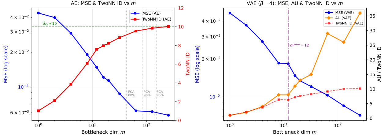
図 3: Exp-Mnist-Base : MNIST における各指標の m 依存性 (300 エポック). 左 (AE) : MSE (対数スケール, 左軸) と TwoNN ID (右軸). 垂直点線は PCA の累積寄与率 80% (43 次元), 90% (86 次元), 95% (152 次元) に対応; 非線形 AE の推定値 (TwoNN \approx 10 ) との差異が明確である. 右 (VAE, \beta = 4 ) : MSE (対数スケール, 左軸), AU (右軸), TwoNN ID (右軸破線). m = 12 ( m^{\text{knee}} ) で AU 増加率が急落 (矢印) し, 有効表現次元の読み取り点となる.
