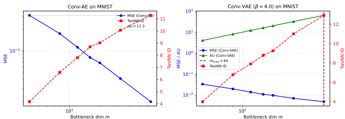
図 9: Exp-Conv-AE : Conv-AE (左) \cdot Conv-VAE (右) における MSE, AU, TwoNN ID の m 依存性 (MNIST, 100 エポック). Conv-AE では \text{AU} = m (全次元活性) が確認され、TwoNN ID が m \geq 32 で \approx 11 に収束する。Conv-VAE では \text{AU} \approx m (100 エポックの収束不足により飽和なし)。
