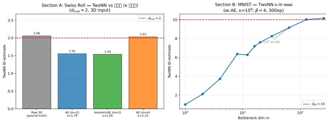
図 2: 実験 Exp-Stab : (左) Swiss Roll での TwoNN ID 棒グラフ – m = d_{\text{true}} = 2 では AE・IsometricAE ともに TwoNN \approx 1.55 ( \kappa 差よりボトルネック余裕の不足が主因) ; m = 4 > d_{\text{true}} で TwoNN が 2.03 へ回復. (右) MNIST VAE TwoNN vs m 収束曲線 (参照 AE, \kappa \approx 10^9 ). 実験 Exp-Geom (AEm スイープ) の結果は表 9 を参照.
