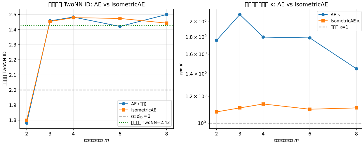
図 3: Exp-Iso-ID : (左) m 別の潜在空間 TwoNN ID— AE (通常) と IsometricAE の曲線はほぼ重なり, 等長性改善による TwoNN ID への影響が軽微であることを示す; (右) デコーダ条件数 \kappa の比較— IsometricAE は全 m で \kappa \approx 1.1 を維持し, AE は m = 3 で \kappa = 2.10 まで上昇する.
