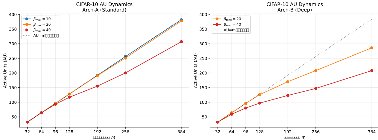
図 15: Exp-NatImg-AU : CIFAR-10 Conv-VAE の AU 動態. (左) Arch-A (Standard), (右) Arch-B (Deep). 点線は \text{AU} = m (飽和なし) の参照線. \beta_{\text{max}} 増大により AU 抑制は強まるが, いずれの条件でも飽和プラトーに至らない.
