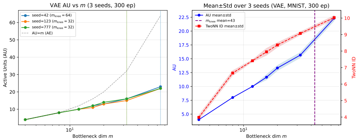
図 6: Exp-Mnist-Multi : MNIST VAE の AU パターン (3 シード, 300 エポック). 左: 各シードの AU vs m (点線は m^{\text{knee}} ); 右: 平均 \pm 標準偏差バンド. AU・TwoNN ID のバンドは非常に狭いが, m^{\text{knee}} はシード間で 32~64 に変動する。
